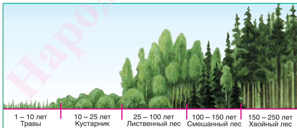
Рис. 36. Схема вторичной сукцессии на месте лесного пожара в умеренном поясе
