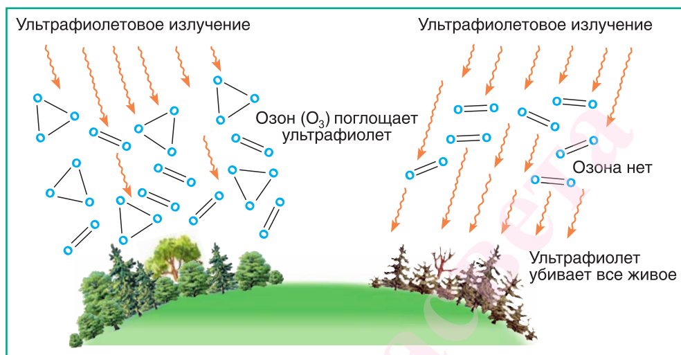
Рис. 91. Защитная роль озона в атмосфере
