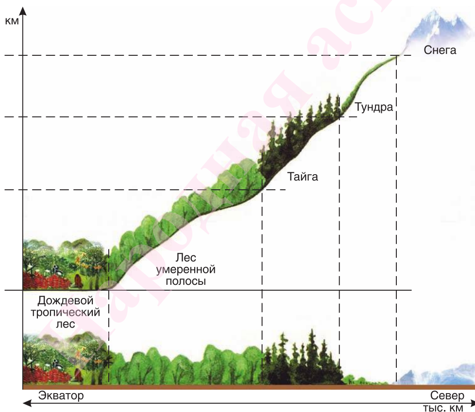
Рис. 15. Смена климатических зон в зависимости от географической широты и высоты в горах
